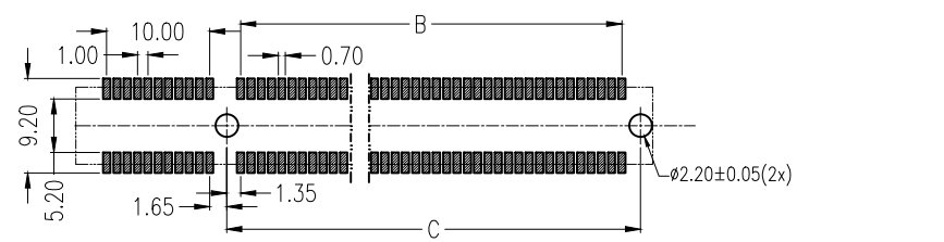
P.C.B LAYOUT(T=1.60mm) COMPONENT SIDE
