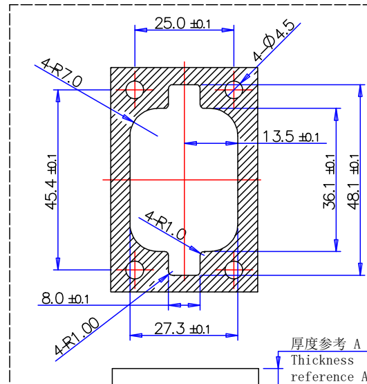
安装板开孔尺寸 Panel Size
