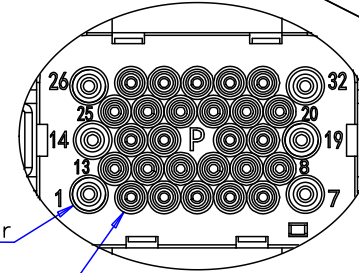
局部视图P Local view P
