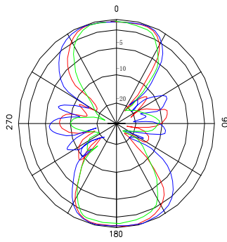
垂直面方向图 Vertical Pattern
