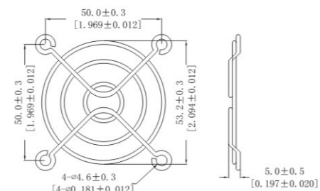
6CM网罩
