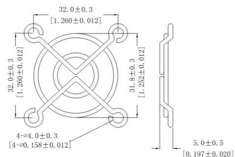
4CM网罩
