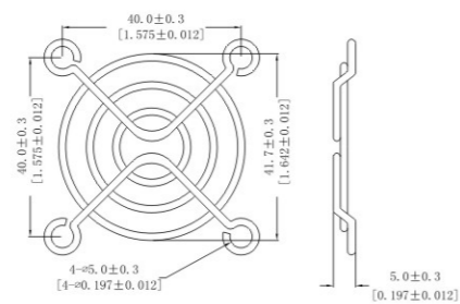
5CM网罩
