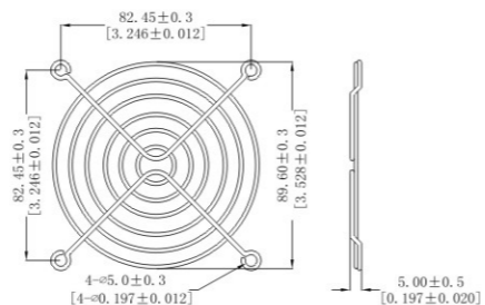
9CM网罩
