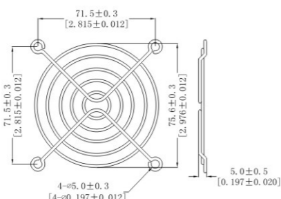
8CM网罩
