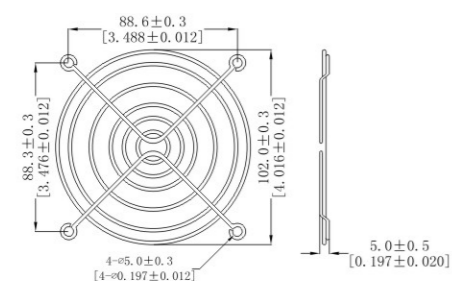
11CM网罩
