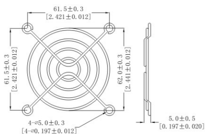
7CM网罩
