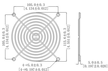
12CM网罩
