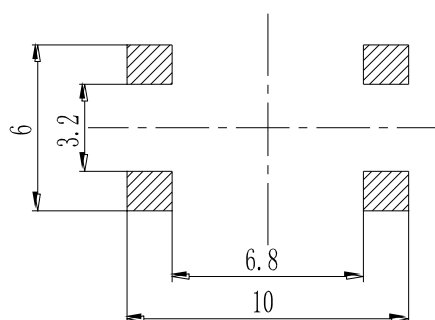
焊接尺寸图:
