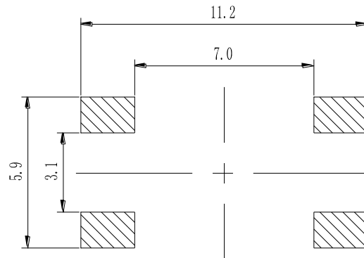
焊接尺寸图
