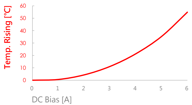
VEFL2C0630-100MPA
