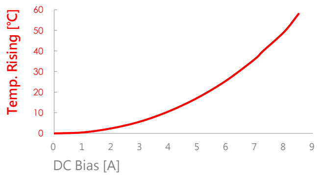
VEFL2C0630-4R7MPA
