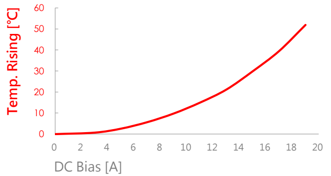
VEFL2C0630-1R0MPA
