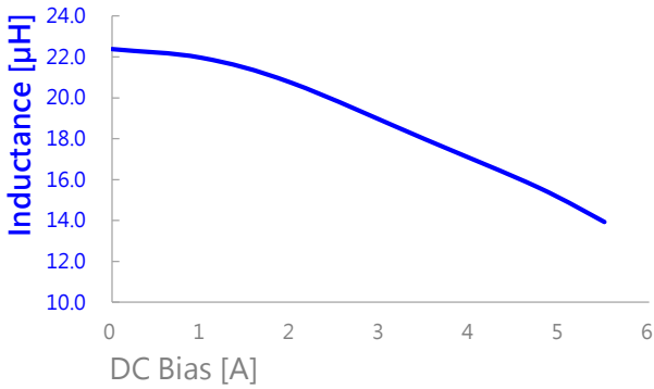
VEFL2C0630-220MPA
