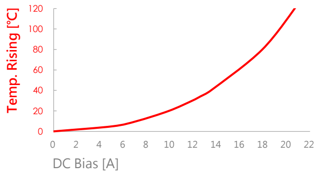
VEFL2C0630-1R5MPA
