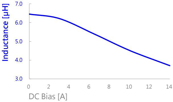
VEFL2C0630-6R8MPA
