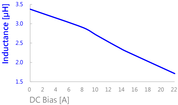
VEFL2C0630-3R3MPA
