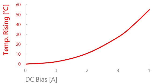
VEFL2C0630-220MPA
