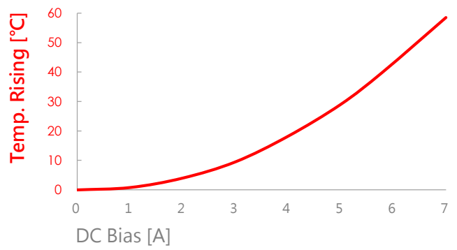
VEFL2C0630-6R8MPA
