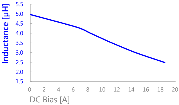
VEFL2C0630-4R7MPA
