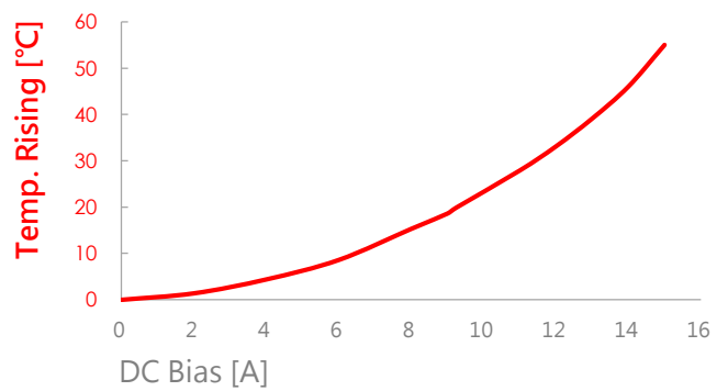
VEFL2C0630-1R8MPA
