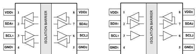
CMT8100 NB SOIC-8
