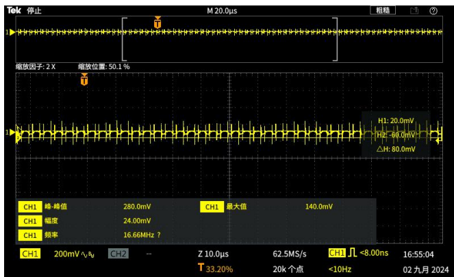
Output ripple (12V /7A)
